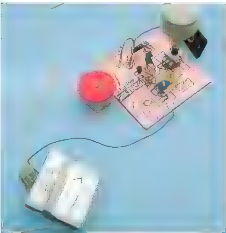
Dit is het proefprintje voor het testen van verschillende oscillatorschakelingen. De afstem-C is die met het rode knopje. De potmeter op de achtergrond dient om de gevoeligheid van de meter te kunnen regelen. De LF-oscillator om te kunnen moduleren is hier nog niet aanwezig.
